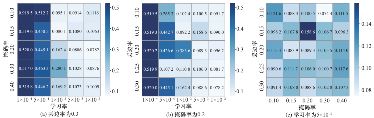
图5 TGMC在不同超参数下的FPR值
