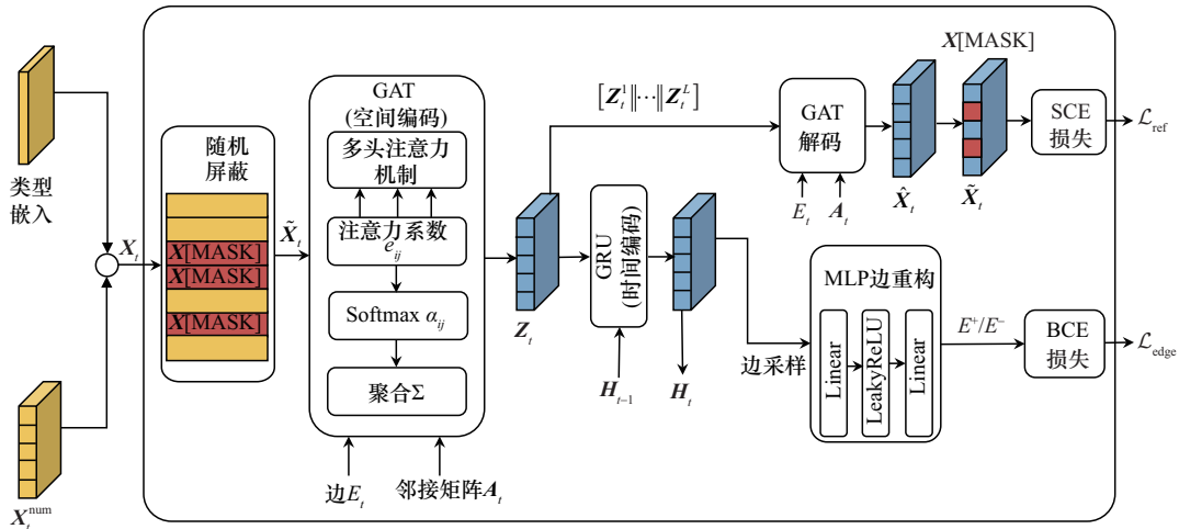
图 2 时空掩码重建
