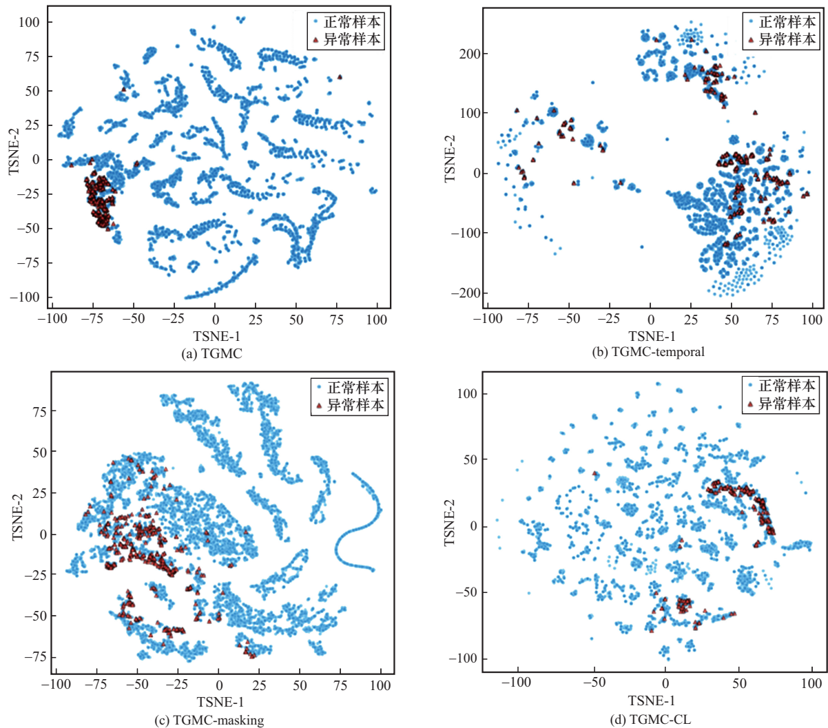
图6 基于CERT r4.2的TSNE可视化结果
