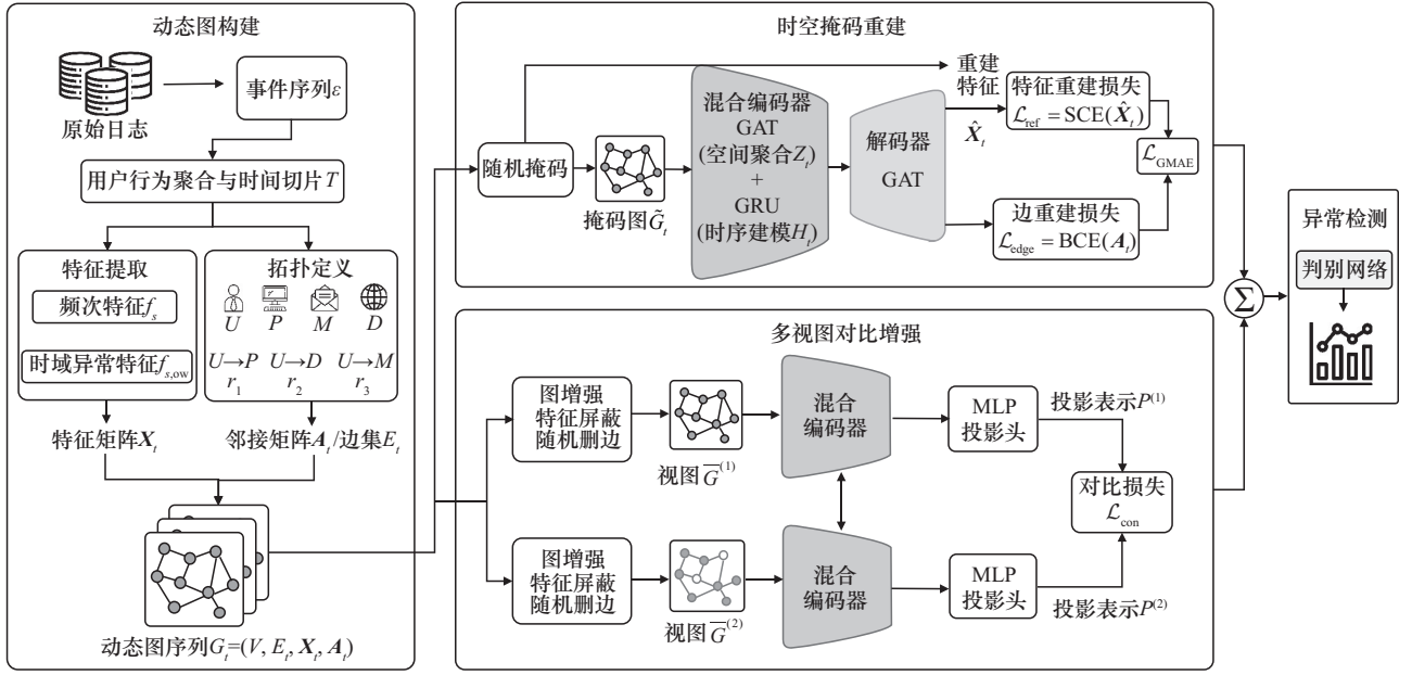
图1 TGMC方法框架
