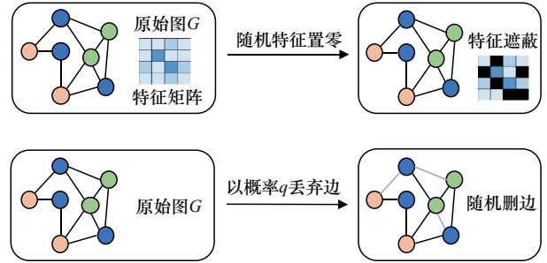
图3 对比视图的扰动策略
