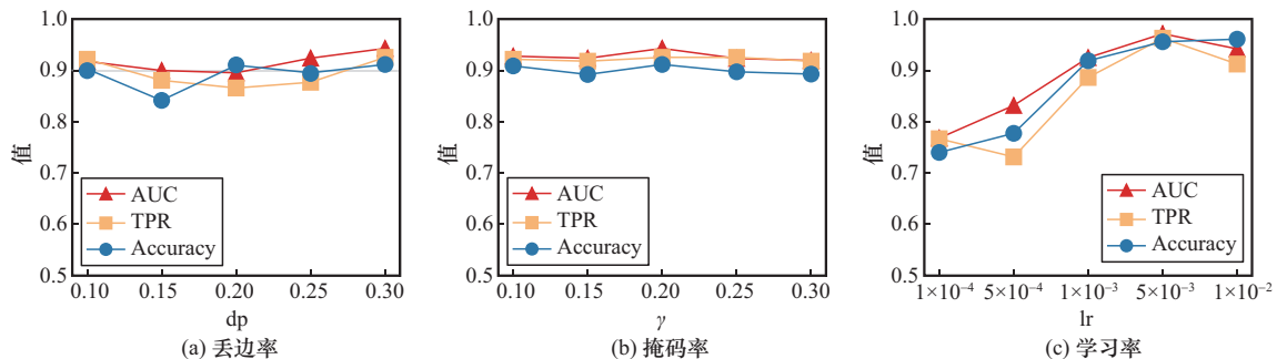
图4 TGMC在不同超参数下的性能
